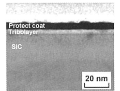
図3 水潤滑において炭化ケイ素表面に自己形成されたナノ界面(Tribolayer)
